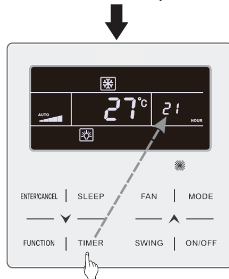
Fig. 4.3 Ajuste de apagado mediante programador con la máquina en estado "ON"
